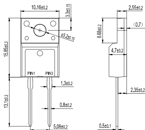
ITO-220AC FR8XXF
