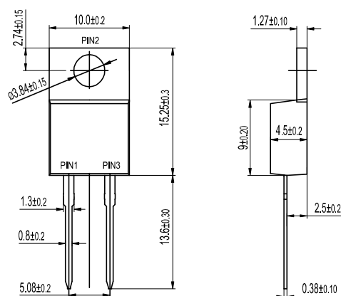
TO-220AC FR8XX
